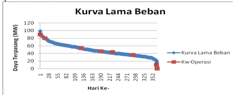
Gambar 6 Kurva Lama Beban
