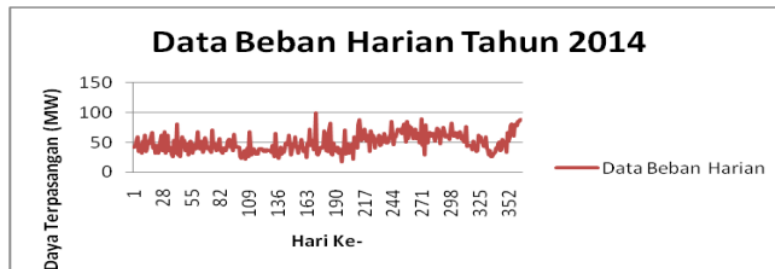
Gambar 5 Kurva Beban Harian Tahun 2014
